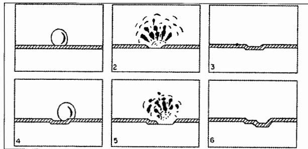
Figura 2. Cavitación. Cuando un líquido fluye a través de una región donde la presión es menor que su presión de vapor, el líquido hierve y forma burbujas de vapor. Estas burbujas son transportadas por el líquido hasta llegar a una región de mayor presión, donde el vapor regresa al estado líquido de manera súbita con implosión brusca de las burbujas, provocando daño en la pared de estructuras cercanas.
