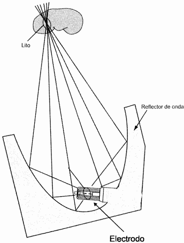
Figura 3. Litotriptor electrohidráulico (primera generación).
