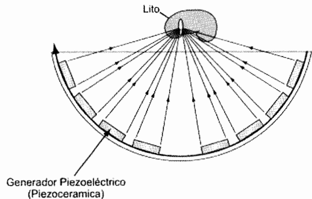
Figura 4. Litotriptor piezoeléctrico (segunda generación).
