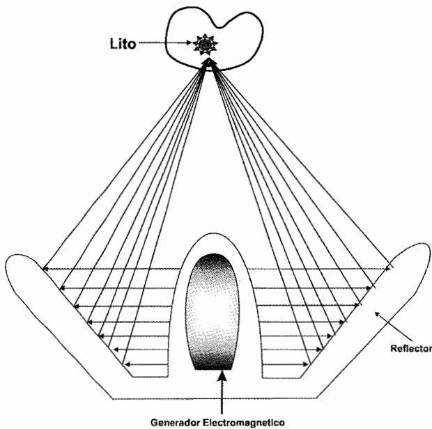
Figura 5. Litotriptor electromagnético (tercera generación).
